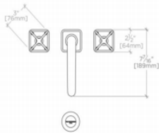
TOP VIEW SCALE: 3/4"=1'-0"
